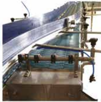
Bant Kaydırıcı Çoklu Nozül Strip Sliding Multiple Nozzle
